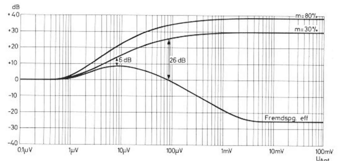
Fremdspannungsverlauf AM in Abhängigkeit von der Antennenspannung
