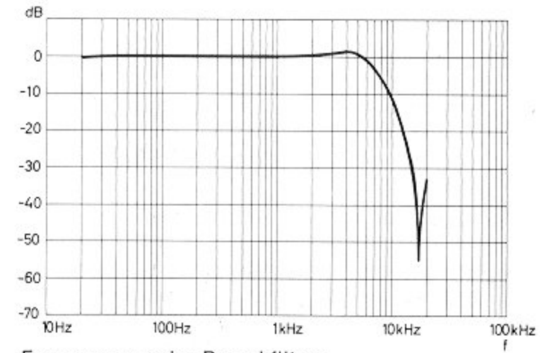
Frequenzgang des Rauschfilters
