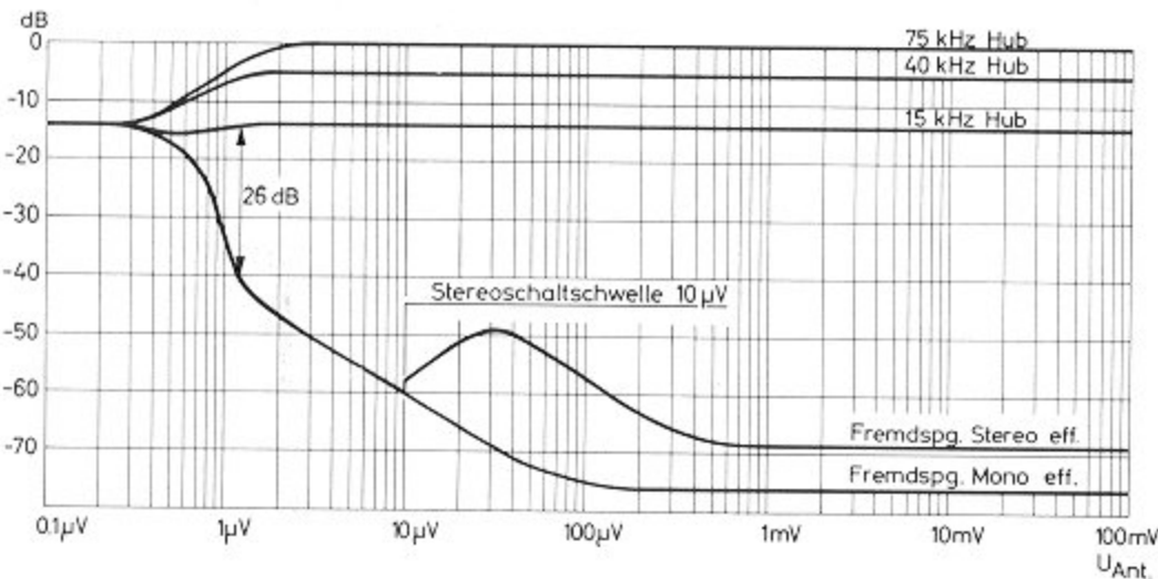
Fremdspannungsverlauf FM in Abhängigkeit von der Antennenspannung
