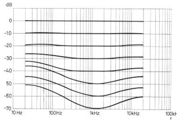
Verlauf der gehörrichtigen Lautstärkekorrektur
