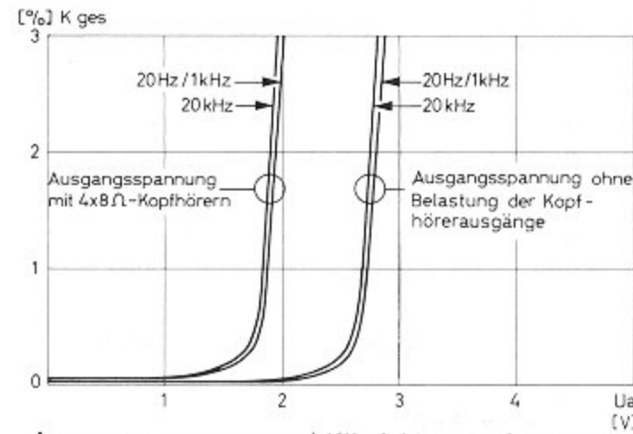
Ausgangsspannung und Klirrfaktor am Ausgang für Aktiv-Boxen (bei 230 V Netzspannung)
